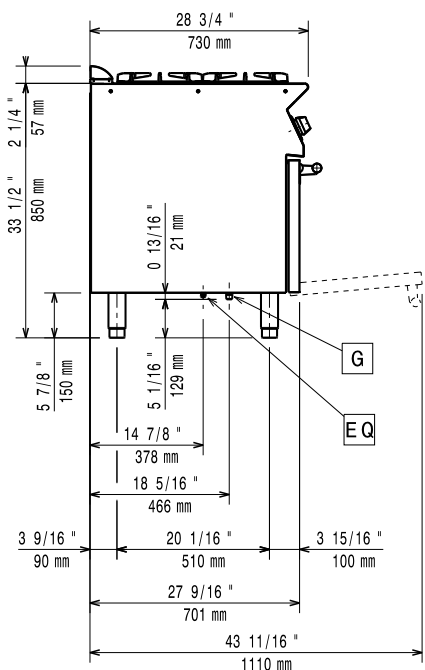
Oldalnézet
